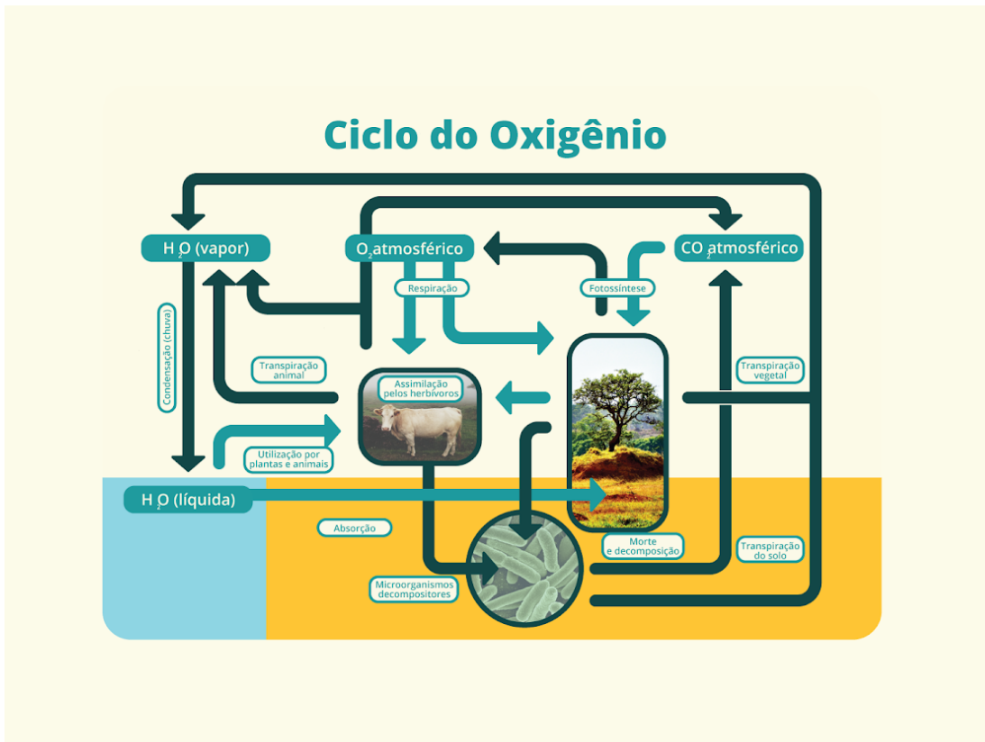
Figura 1. Fatores que contribuem com o equilíbrio na Terra
