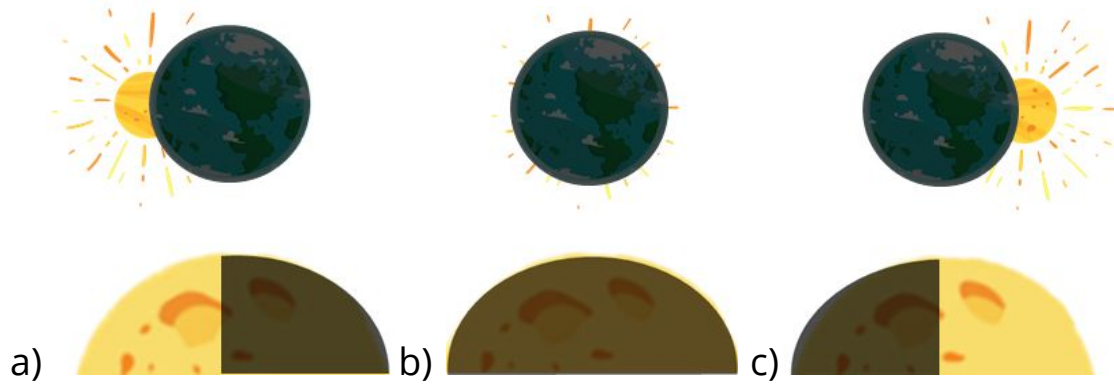
Figura 1. O eclipse lunar visto da Lua em três momentos (a-c). Movimento aparente do Sol sendo: a) parcialmente ocultado pela Terra; b) completamente ocultado pela Terra; c) parcialmente ocultado pela Terra. Este esquema não está em escala.
