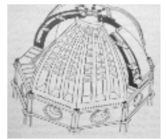
Corte cúpula segundo Heydenreich e Lotz
