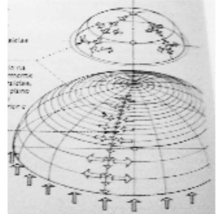
Corte cúpula segundo Heydenreich e Lotz
