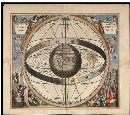
Fig. 1 SISTEMA DE PTOLOMEU - O GEOCENTRISMO
