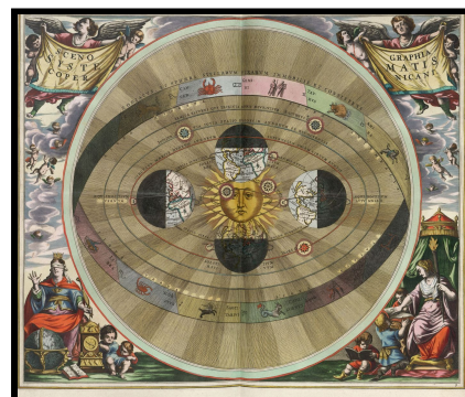
Fig. 2 SISTEMA DE COPÉRNICO - O HELIOCENTRISMO
